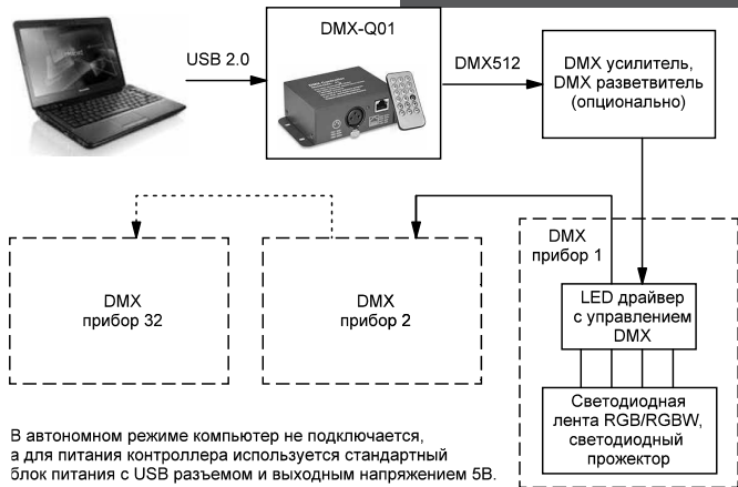
Рис. 4. Структурная схема подключения.
