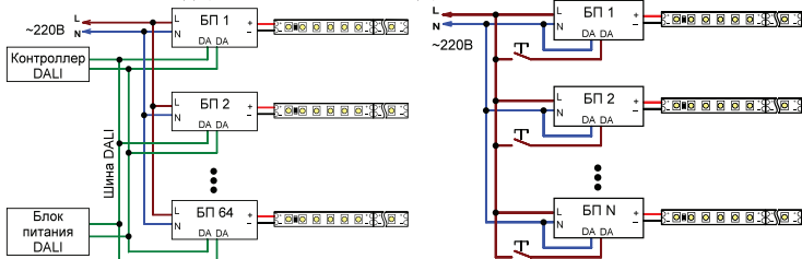
Рис.2. Структурная схема подключения оборудования при использовании интерфейса DALI.
