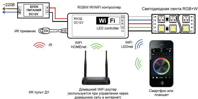
Рис.1. Схема подключения.
