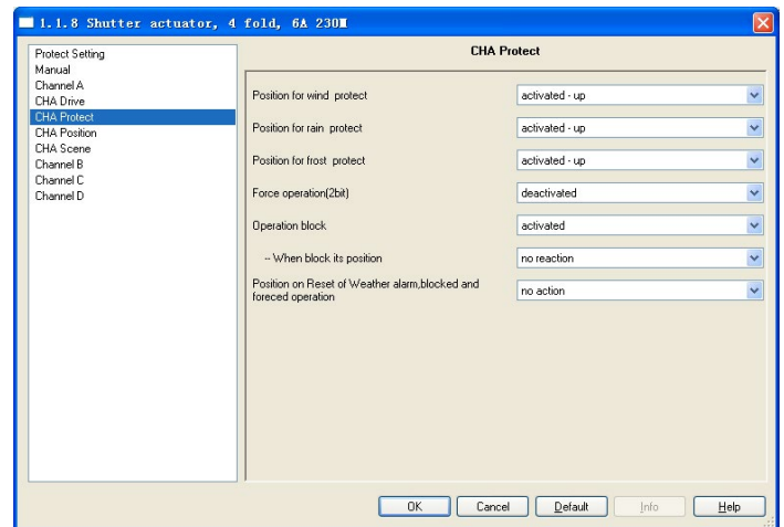
Fig. 3.5 parameter window "CHA Protect"
