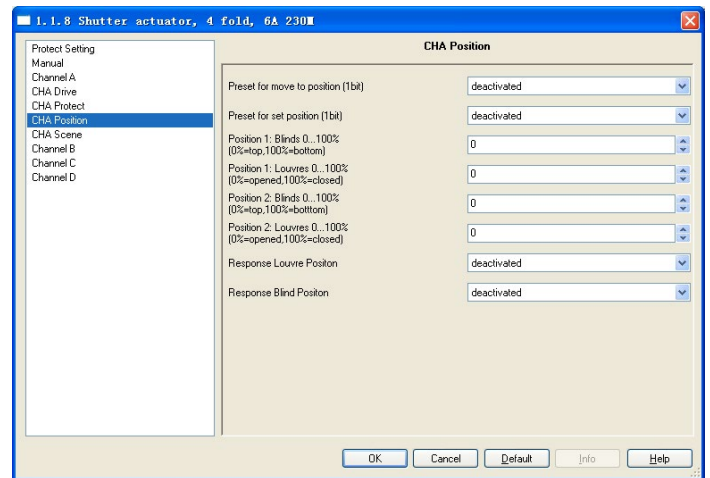
Fig. 3.6 parameter window "CHA Position"
