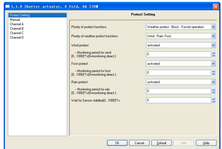
Fig.3.1 parameter window "Protect Setting"
