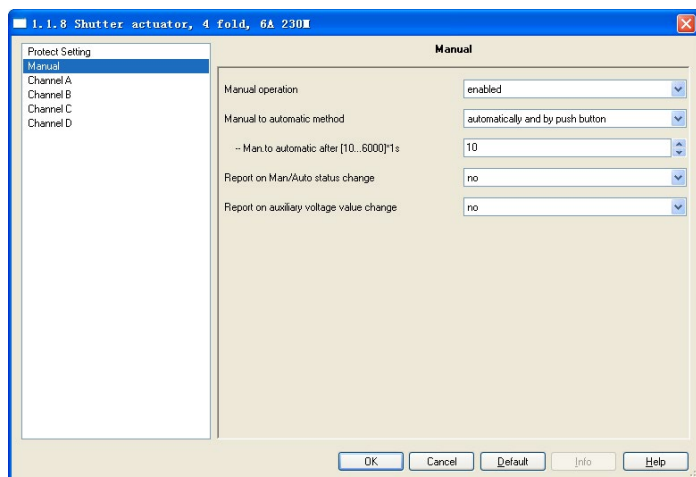
Fig.3.2 parameter window "manual"
