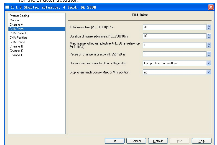
Fig.3.4 parameter window "CHA Drive"
