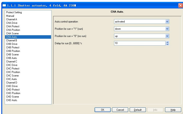
Fig. 3.8 parameter window "CHA Auto."
