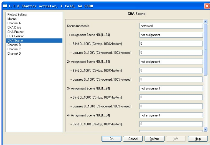
Fig. 3.7 parameter window "CHA Scene"
