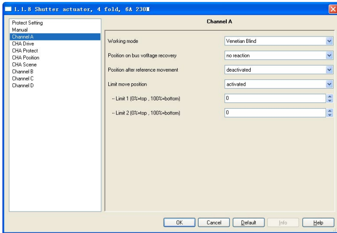
Fig. 3.3 parameter window "Channel X"
